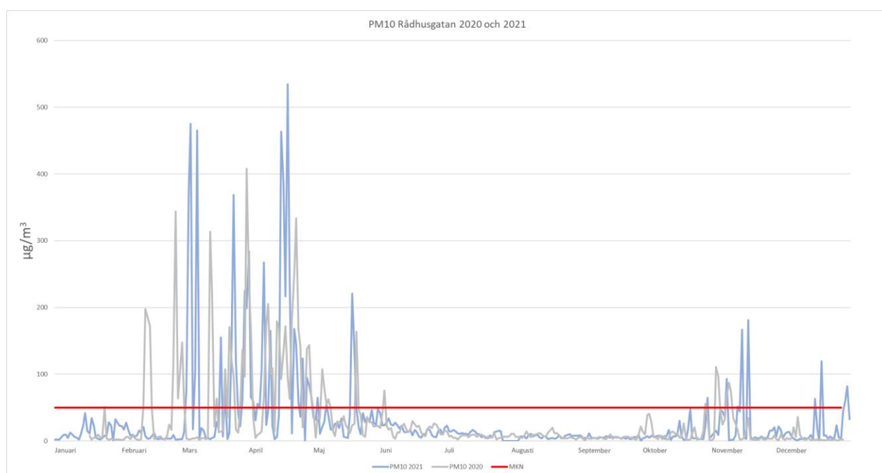
Figur 4. Uppmätta halter av PM10 på Rådhusgatan under 2020 och 2021, jämförelse mot miljö kvalitetsnorm, MKN. Kvalitetssäkrade data.
