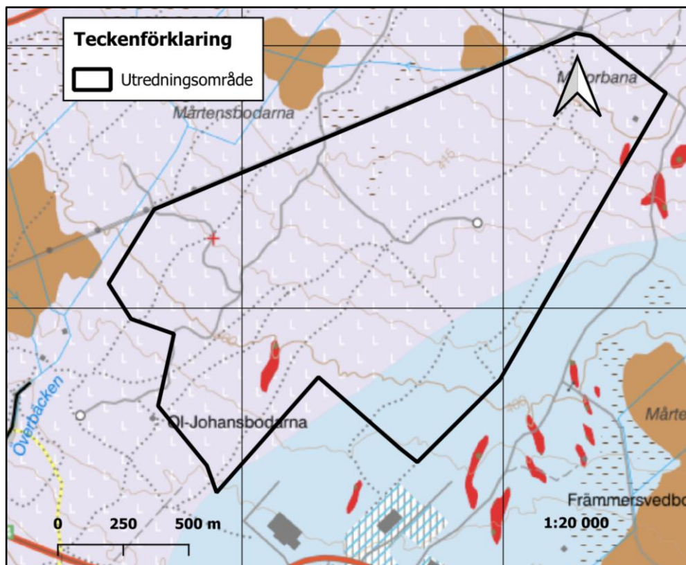
Figur 4. SGU (2024-05-28) redovisar det lösa jordtäcket i utredningsområdet som moränlera Ljus violett med stående L. I sydost över går moränleran i moränmark (ljusblått). Inslag av torv (streck) och hållmark förekommer. SGU:s kartering avser förhållanden på 0,5 meters djup under markytan. Skala 1:20 000.
