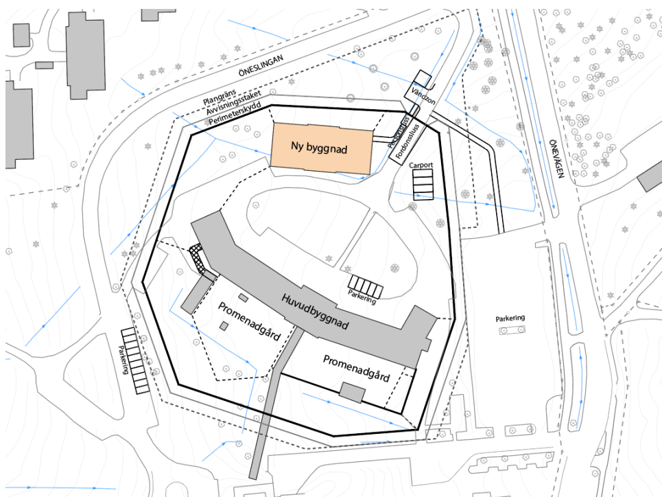
Illustration över planområdet där placering av ny byggnad samt verksamhetsspecifika behov illustrerats. Plangränsen (streckad linje).
