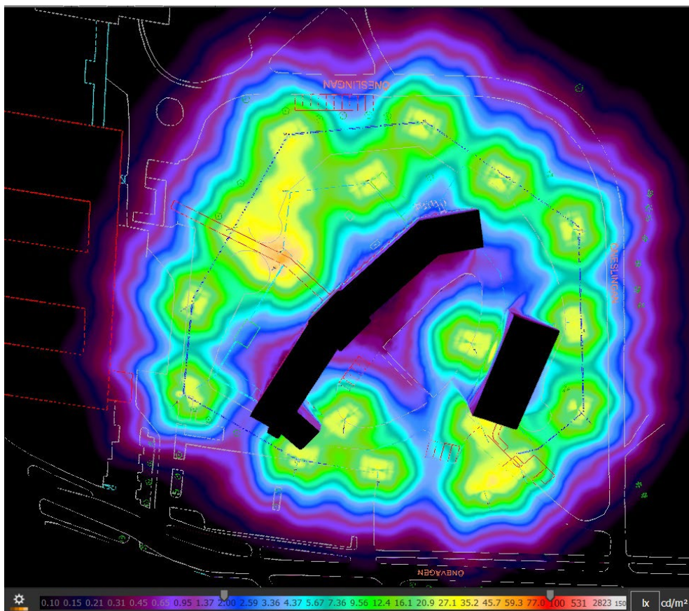
Falskfärgbild över ljusets utbredning i området. Siffrorna är i enheten Lux. Den mörkblå linjen som ligger en bit ifrån perimeterskyddet är linjen för gränsvärdet 2 lux.
