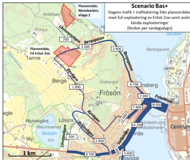
Figur 23. Trafikflöden i scenario Bas+ med full exploatering av Frösö Zoo. Bildkälla: Lantmäteriet, bearbetad av Sigma Civil
