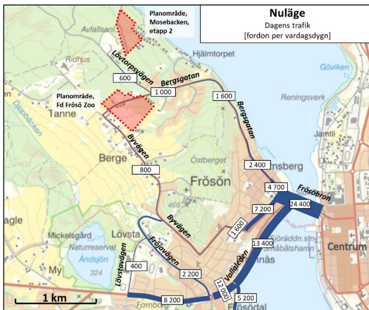
Figur 20. Trafikflöden för nuläget. Bildkälla: Lantmäteriet, bearbetad av Sigma Civil
