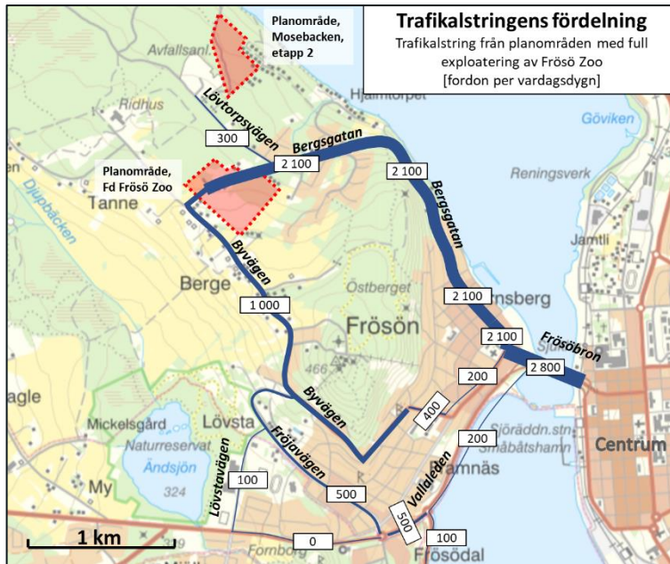
Figur 19. Den alstrade trafikens spridning i vägnätet. Bildkälla: Lantmäteriet, bearbetad av Sigma Civil
