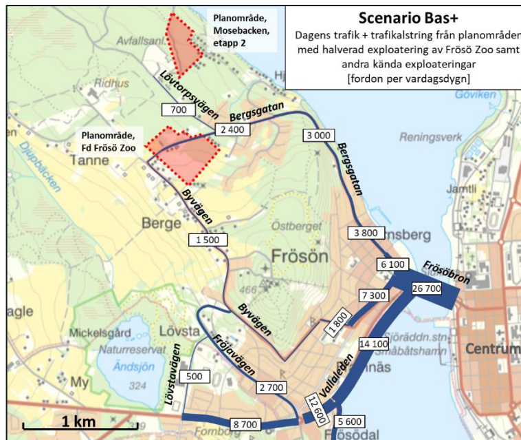
Figur 24. Trafikflöden i scenario Bas+ med halverad exploatering av Frösö Zoo. Bildkälla: Lantmäteriet, bearbetad av Sigma Civil
