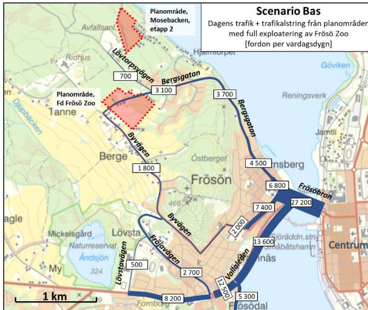
Figur 21. Trafikflöden i scenario Bas med full exploatering av Frösö Zoo. Bildkälla: Lantmäteriet, bearbetad av Sigma Civil
